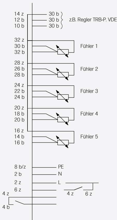
Steckerbelegung z und d
